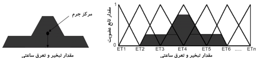
شکل ۳- نافازی سازی خروجی مدل با روش مرکز ثقل
