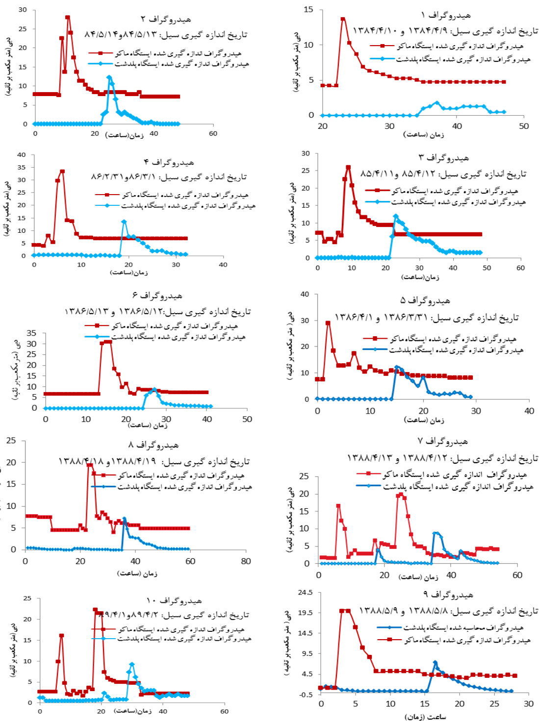
شکل ۲- هیدروگراف های سیل اندازه گیری شده در ایستگاه های ماکو و پلدشت
