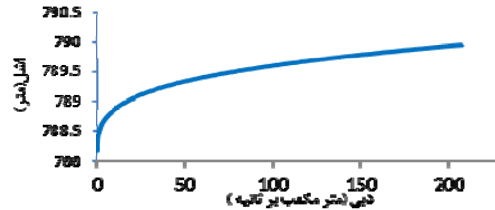
شکل ۶- رابطه دبی - اشل ایستگاه هیدرومتری پلدشت
