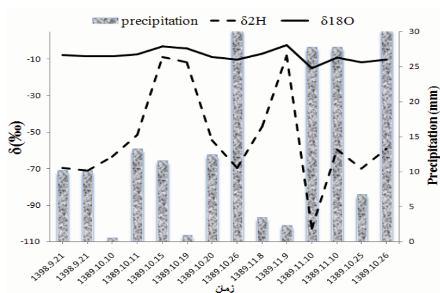
شکل ۴- ارتباط بین میزان بارندگی و مقادیر \delta^2\text{H} و \delta^{18}\text{O} نمونه‌های باران
