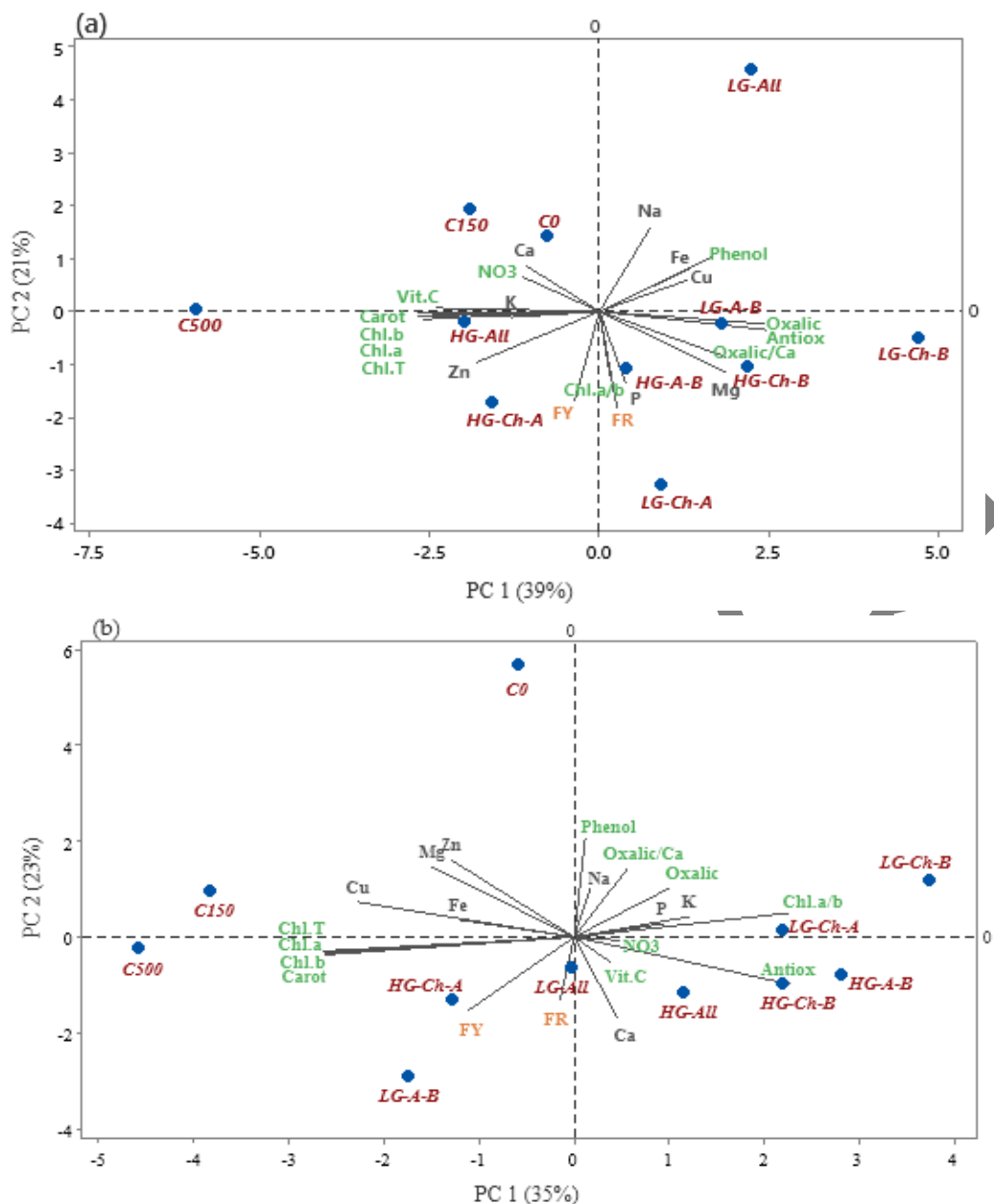
شکل ۱- تجزیه مولفه‌های اصلی (PCA) داده‌های گیاه (عناصر غذایی، ویژگی‌های فیزیولوژیک، و وزن تازه بخش هوایی (FY) و وزن تازه ریشه (FR) برای کشت اول (a) و کشت دوم (b). برای علائم اختصاری تیمارها به جدول ۴ مراجعه کنید.
