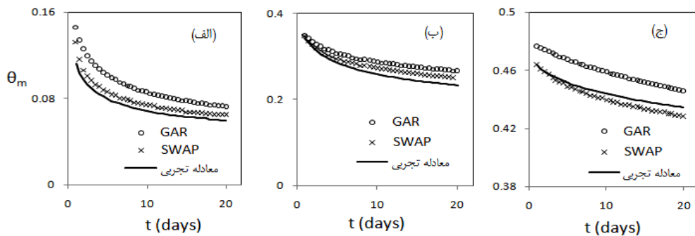
(شکل ۱۳) - تغییرات زمانی درصد رطوبت میانگین جبهه رطوبتی در بافت (الف) شن، (ب) لوم و (ج) رس برای عمق آب نفوذ یافته 100mm و مکش یکنواخت خاک پیش از نفوذ 10 5 cm. به دست آمده از خروجی‌های مدل های GAR، SWAP و معادله تجربی پیشنهادی.
