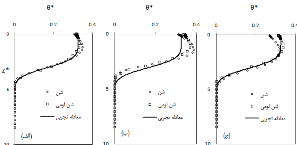
(شکل ۷) - نیمرخ رطوبت مقیاس شده خاک‌های درشت بافت در زمان مقیاس شده (الف) t^*=100 ، (ب) t^*=200 و (ج) t^*=300 برای عمق آب نفوذ یافته mmI=100 و مکش یکنواخت خاک پیش از نفوذ h_i=10^5 \text{ cm} . نقاط مربوط به خروجی‌های SWAP می‌باشند.
