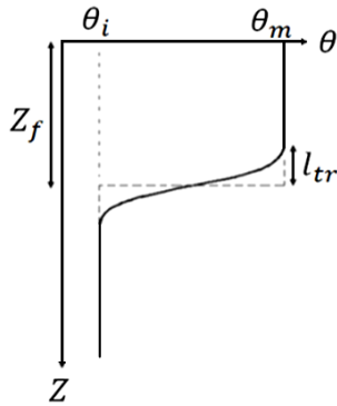
(شکل ۳) - شرح ترسیمی پارامترهای معادله تجربی پیشنهادی.
