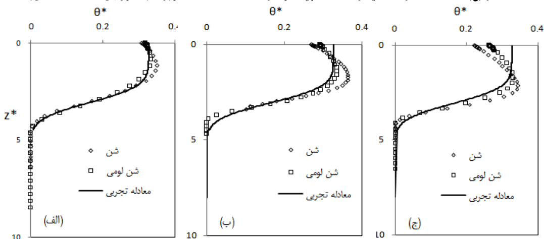
(شکل ۹) - نیمرخ رطوبت مقیاس شده خاک‌های ریز و متوسط بافت در زمان مقیاس شده t^*=1 برای عمق آب نفوذ یافته (الف) mmI=100 (ب) و mmI=200 (ج) و مکش یکنواخت خاک پیش از نفوذ h_i=10^5 cm . نقاط مربوط به خروجی‌های SWAP می‌باشند.
