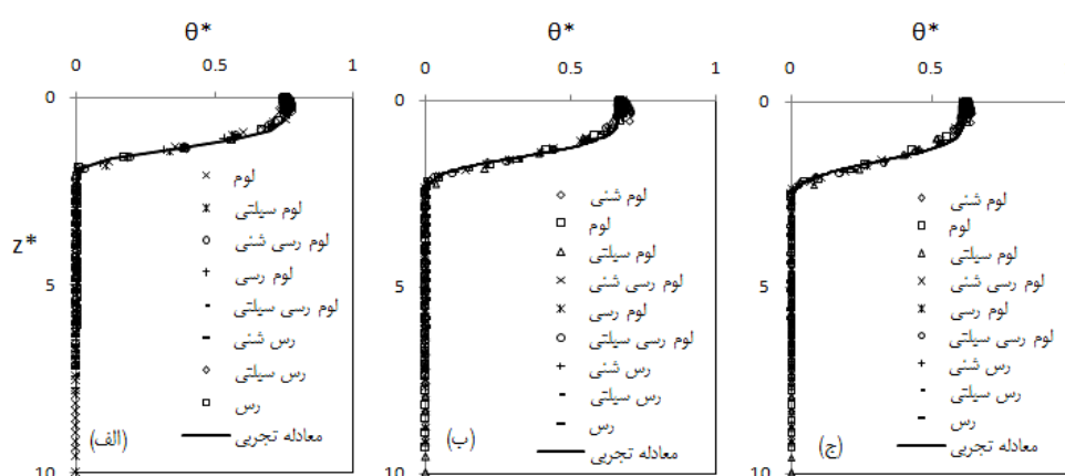
(شکل ۶) - نیمرخ رطوبت مقیاس شده خاک‌های ریز و متوسط بافت در زمان مقیاس شده (الف) t^*=1 ، (ب) t^*=3 و (ج) t^*=5 برای عمق آب نفوذ یافته mmI=100 و مکش یکنواخت خاک پیش از نفوذ h_i=10^5 \text{ cm} . نقاط مربوط به خروجی‌های SWAP می‌باشند.
