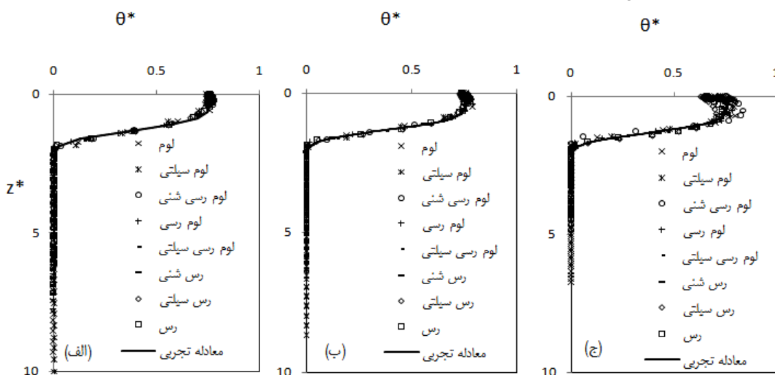
(شکل ۱۱) - نیمرخ رطوبت مقیاس شده خاک‌های ریز و متوسط بافت در زمان مقیاس شده t^*=100 برای عمق آب نفوذ یافته mmI=100 و مکش یکنواخت خاک پیش از نفوذ (الف) h_i=10^5\text{cm} ، (ب) h_i=10^4\text{cm} و (ج) h_i=10^3\text{cm} . نقاط مربوط به خروجی‌های SWAP می‌باشند.
