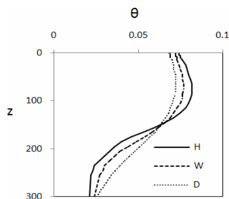
(شکل ۵) - تأثیر پس‌ماند بر فرآیند توزیع مجدد در یک خاک شنی. نیمرخ رطوبت خاک با وجود پس‌ماند (H) با شرایطی که پس‌ماند وجود ندارد مقایسه شده است. W نشان دهنده خاک بدون پس‌ماند بر پایه شاخه خیس‌شدگی منحنی رطوبتی و D نشان دهنده خاک بدون پس‌ماند بر پایه شاخه خشک‌شدگی منحنی رطوبتی می‌باشد.
