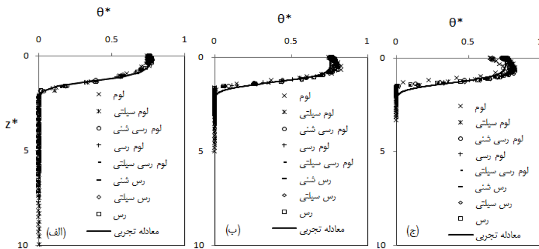
(شکل ۹) - نیمرخ رطوبت مقیاس شده خاک‌های ریز و متوسط بافت در زمان مقیاس شده t^*=1 برای عمق آب نفوذ یافته (الف) mmI=100 (ب) و mmI=200 (ج) و مکش یکنواخت خاک پیش از نفوذ h_i=10^5 cm . نقاط مربوط به خروجی‌های SWAP می‌باشند.
