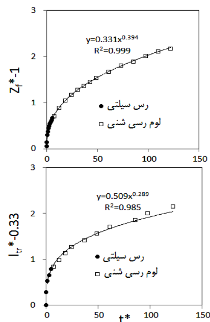
(شکل ۴) ارتباط تابعی بین z_f^* و l_{ir}^* با زمان مقیاس شده ( t^* ).
