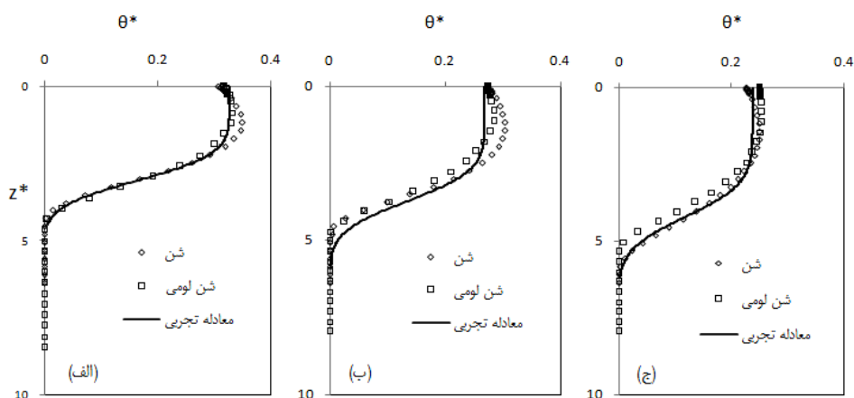
(شکل ۷) - نیمرخ رطوبت مقیاس شده خاک‌های درشت بافت در زمان مقیاس شده (الف) t^*=100 ، (ب) t^*=200 و (ج) t^*=300 برای عمق آب نفوذ یافته mmI=100 و مکش یکنواخت خاک پیش از نفوذ h_i=10^5 \text{ cm} . نقاط مربوط به خروجی‌های SWAP می‌باشند.
