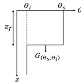
(شکل ۱) - شرح ترسیمی پارامترهای مدل نفوذ گرین-امپت.
