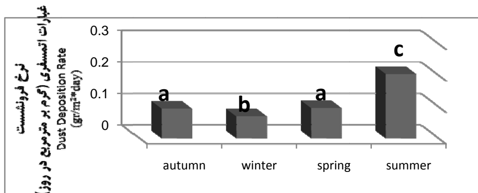
شکل ۲- نمودار نرخ فرونشست غبارات اتمسفری در فصول سال (حروف متفاوت، نشان‌دهنده تفاوت معنی‌دار در سطح ۹۹ درصد هستند).
