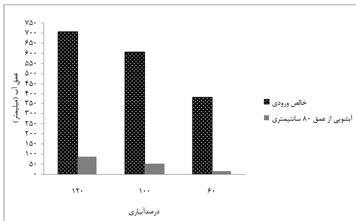
شکل ۳- مقادیر آب خالص داده شده و نفوذ عمقی آب در تیمارهای سطوح آبی ۶۰، ۱۰۰ و ۱۲۰ درصد
