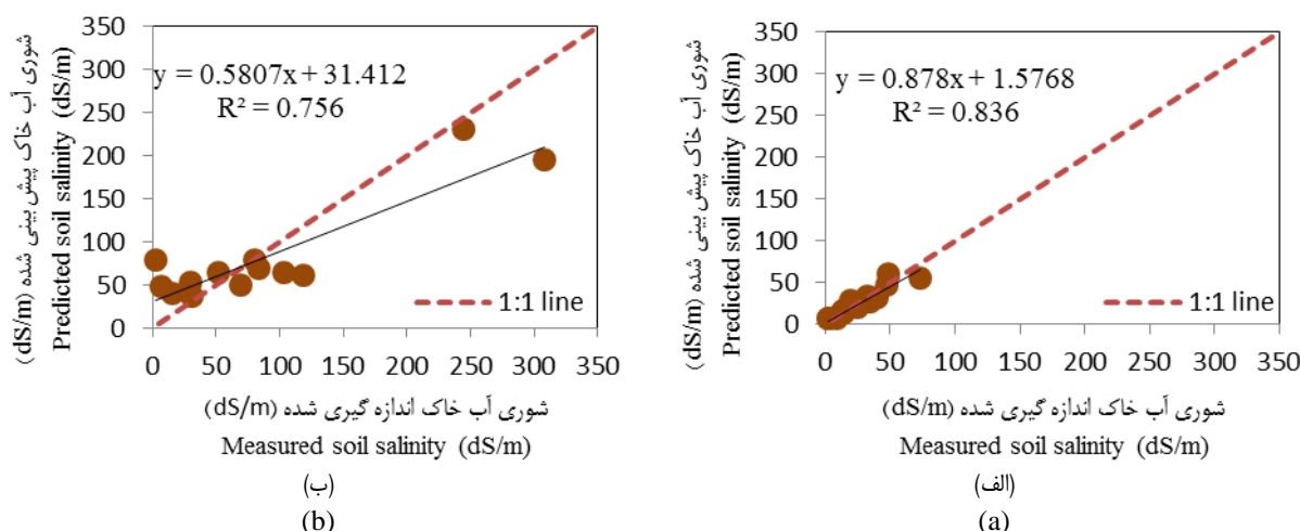
شکل ۵- مقادیر پیش‌بینی شوری خاک با استفاده از طیف‌های جذبی به وسیله مدل PLSR در بافت خاک (الف) سنگین و (ب) سبک Figure 5- Predicted soil salinity using of absorbance spectra using PLSR model in soil textures of a) coarse and b) fine
