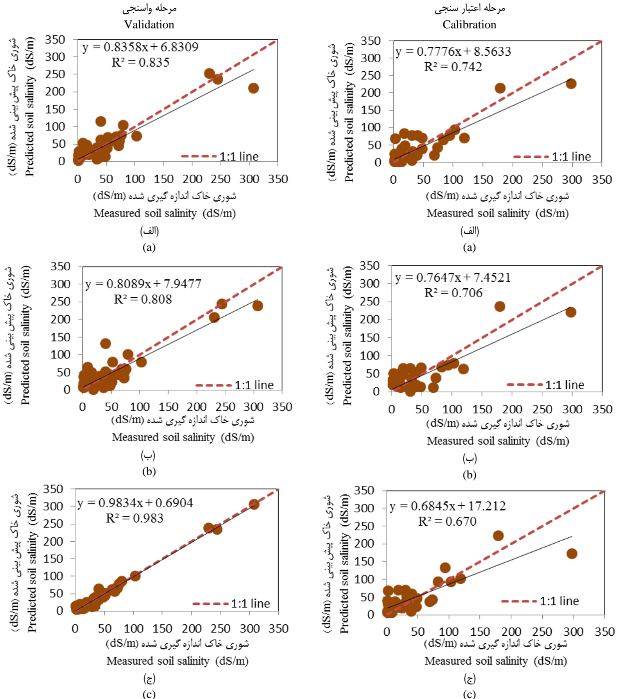
شکل ۴- مقادیر پیش‌بینی شده و اندازه‌گیری شده شوری خاک در مراحل واسنجی و اعتبار سنجی به وسیله مدل PLSR با استفاده از الف) طیف‌های جذبی، ب) طیف‌های بازتابی و ج) مشتق اول طیف بازتابی
