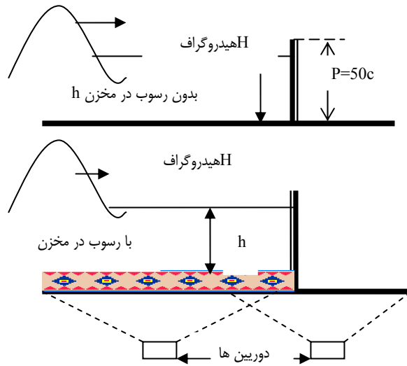
(شکل ۲) - ورود هیدروگراف به کانال و موقعیت دوربین ها
