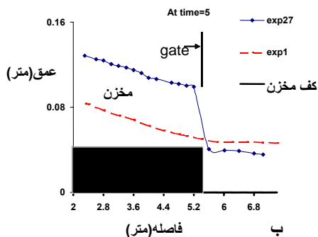
(شکل ۴) - تغییرات تراز سطح آب در حالت بدون هیدروگراف با وبدون رسوب در دو زمان انتخابی ۵ و ۴ برای \frac{h}{p} = 0.2
