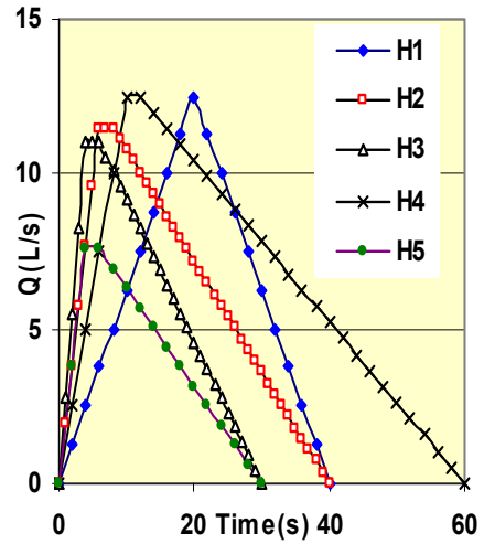
(شکل ۱) - نمونه هیدروگرافهای تولیدی
