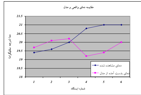
(شکل ۷) - نمودار مقایسه دمای واقعی و مدل روز سوم (ترسیم شده با استفاده از خروجی منطقه)
