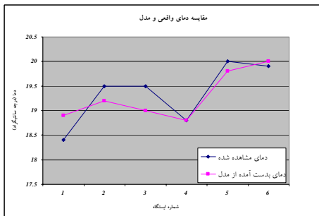
(شکل ۸) - نمودار مقایسه دمای واقعی و مدل روز چهارم (ترسیم شده با استفاده از خروجی منطقه)
