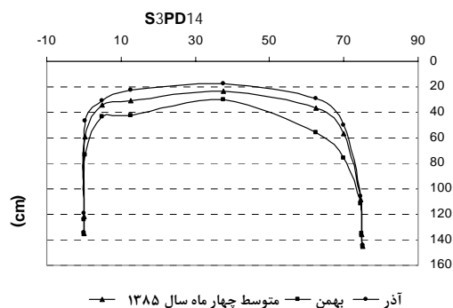
(شکل ۵) - میانگین پروفیل سطح آب زیرزمینی بین دو زهکش S3PD15 و S3PD14 در ماه های آذر (به عنوان بیشترین عمق)، بهمن (به عنوان کمترین عمق) و چهار ماه سال ۱۳۸۵
