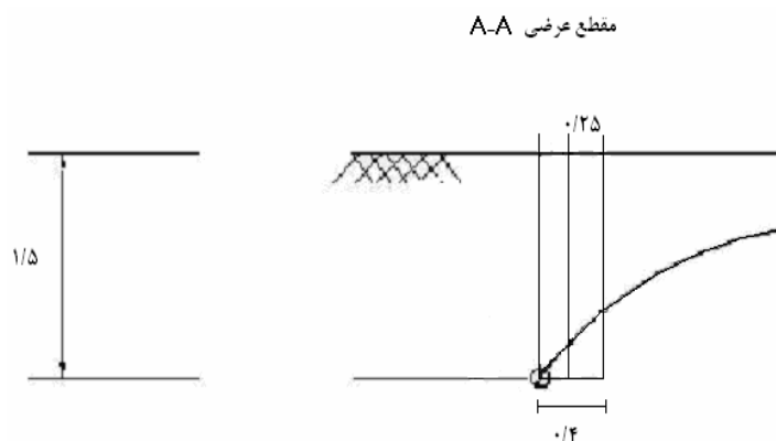
(شکل ۲) - محل نصب پیژومترها در مجاورت زهکش S3PD15 (ابعاد بر حسب متر)
