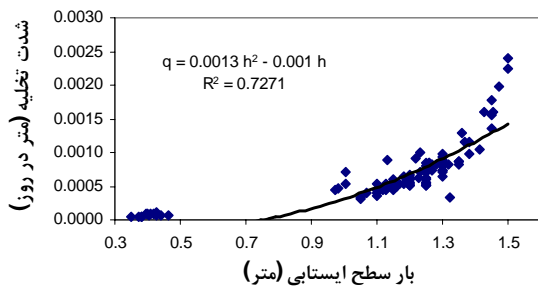
(شکل ۱۱) - رابطه دبی زهکش در مقابل بار سطح ایستابی برای چهار ماه سال ۱۳۸۵، سه ماه سال ۱۳۸۳ و کل داده‌های دو سال
