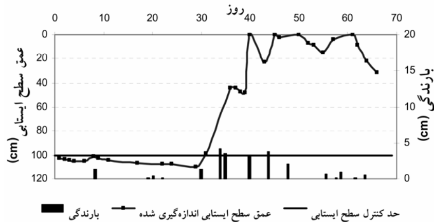
(شکل ۴) - نوسانات سطح ایستابی (در وسط فاصله بین دو زهکش) و بارندگی در ماه‌های مهر، آبان و آذر سال ۱۳۸۳
