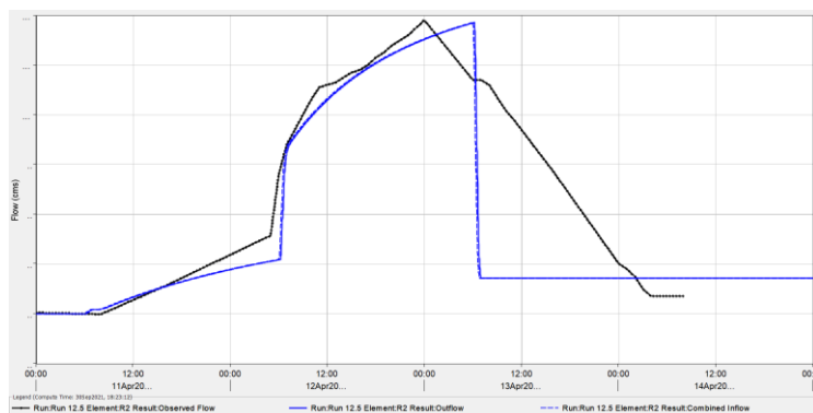
شکل ۱۰- هیدروگراف واقعه ۱۳۹۹/۱/۲۳ Figure 6- Event Hydrograph 23/1/1399
