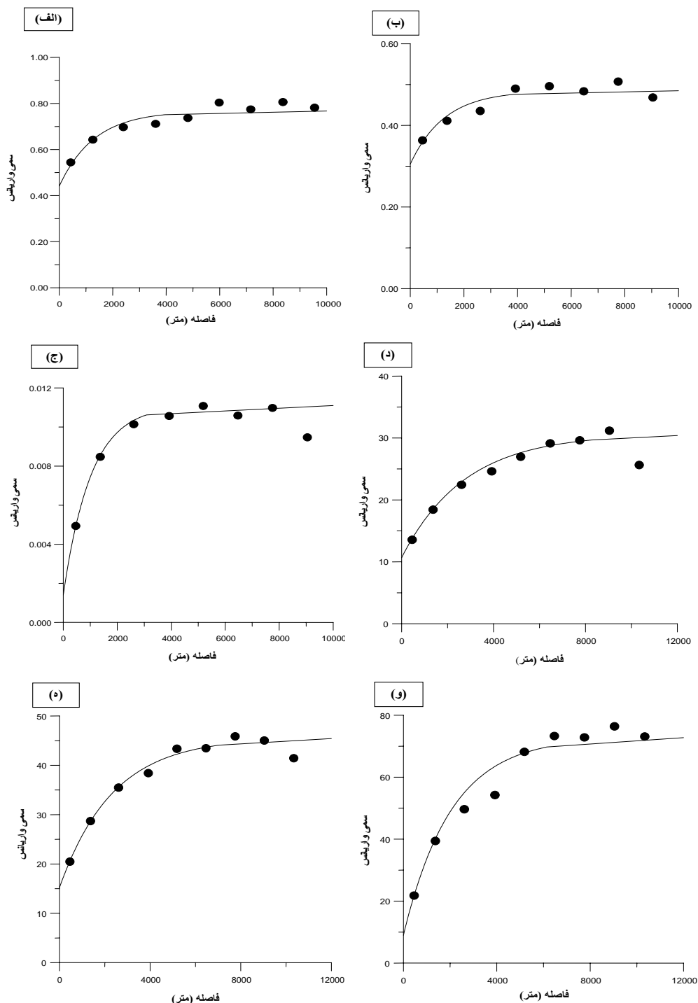
(شکل ۲) - تغییرنماهای همه جهت‌های سرعت نفوذ (الف)، هدایت هیدرولیکی اشباع (ب)، چگالی ظاهری (ج)، درصد رس (د)، درصد سیلت (ه) و درصد شن (و).
