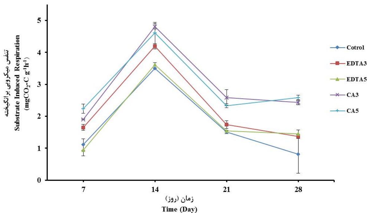
شکل 6- تغییرات SIR خاک در اثر کاربرد EDTA و اسیدسیتریک با گذشت زمان انکوباسیون
