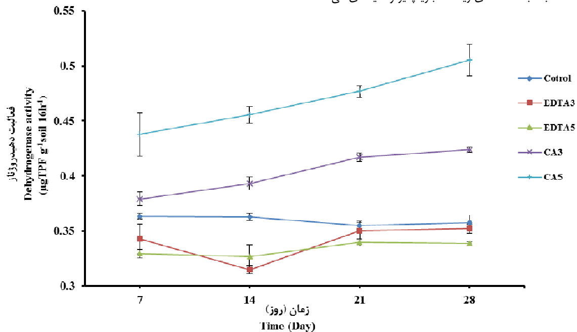
شکل 2- تغییرات فعالیت آنزیم دهیدروژناز خاک در اثر کاربرد EDTA و اسیدسیتریک با گذشت زمان انکوباسیون Figure 2- The effects of EDTA and citric acid on dehydrogenase activity with incubation time
