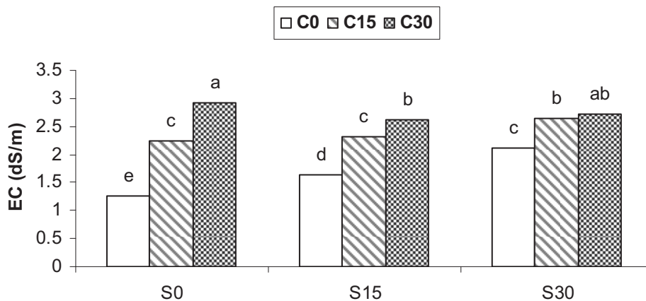
شکل ۸- اثر متقابل سطوح کمپوست پسماند شهری و لجن فاضلاب بر EC خاک C (کمپوست پسماند شهری)، S (لجن فاضلاب) و صفر و ۱۵ و ۳۰ سطوح مختلف کمپوست و لجن فاضلاب می باشند.
