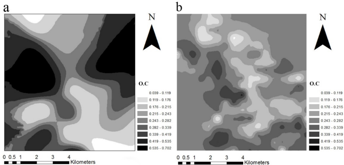
شکل ۳- نقشه پهنه بندی کربن آلی (a) به روش ANN-Kriging و (b) روش کوکرپچینگ
