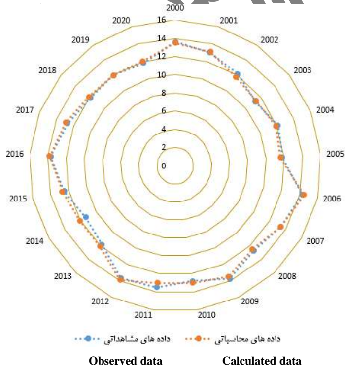
شکل ۶- میانگین سالانه دمای کمینه شهر کرمان، (الف) از ۱۰ مارس تا ۳۱ مارس، (ب) ماه آوریل، (پ) از اول تا ۲۰ می (ترسیم توسط پژوهشگر)
