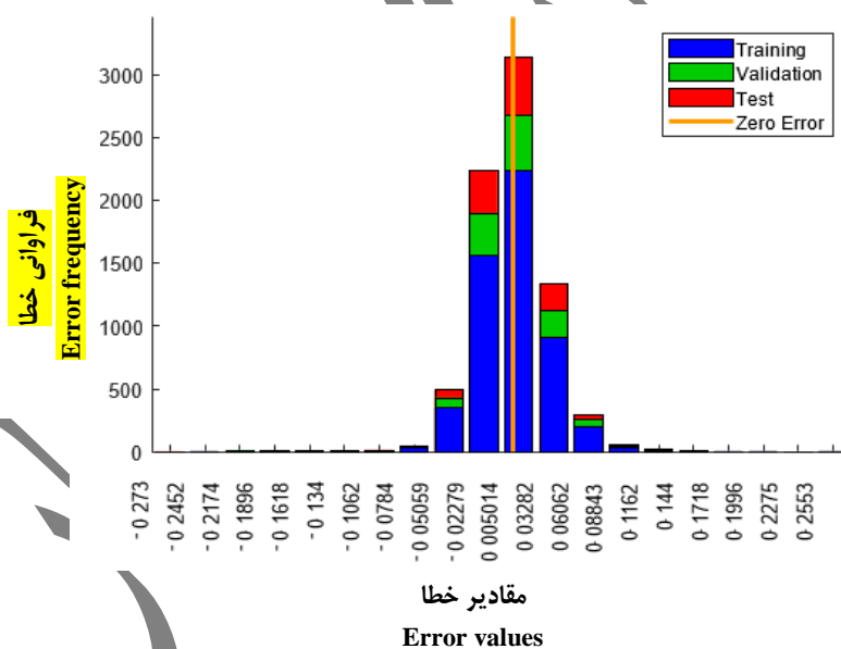
شکل ۴- نمایش مقادیر فراوانی خطای شبکه FFBP در مراحل آموزش، صحت‌سنجی و آزمون (ترسیم توسط پژوهشگر)
