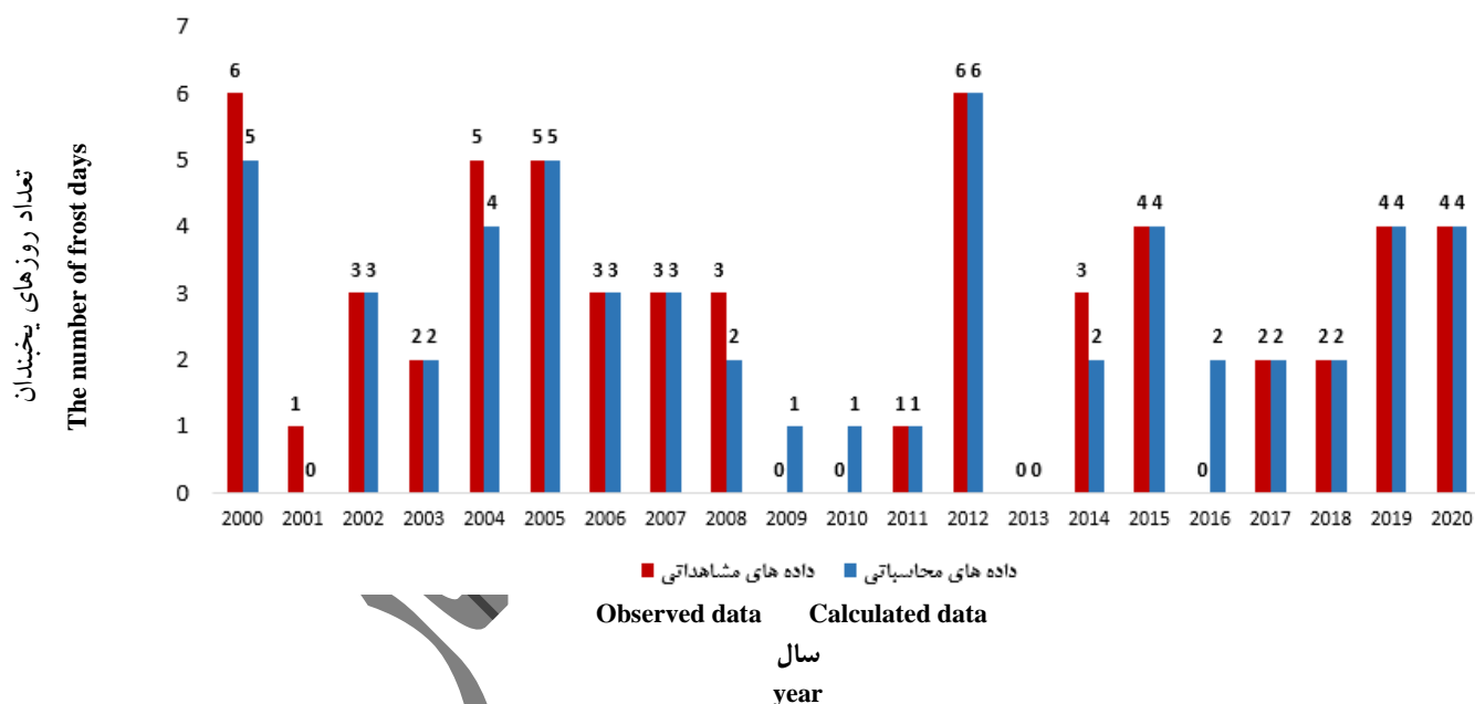
شکل ۷- محاسبه تعداد روزهای یخبندان بهاره در طی سال‌های ۲۰۰۰-۲۰۲۰ (ترسیم توسط پژوهشگر) Figure 7- Calculation of the number of frost days during the years 2000 to 2020 (Created by the author)
