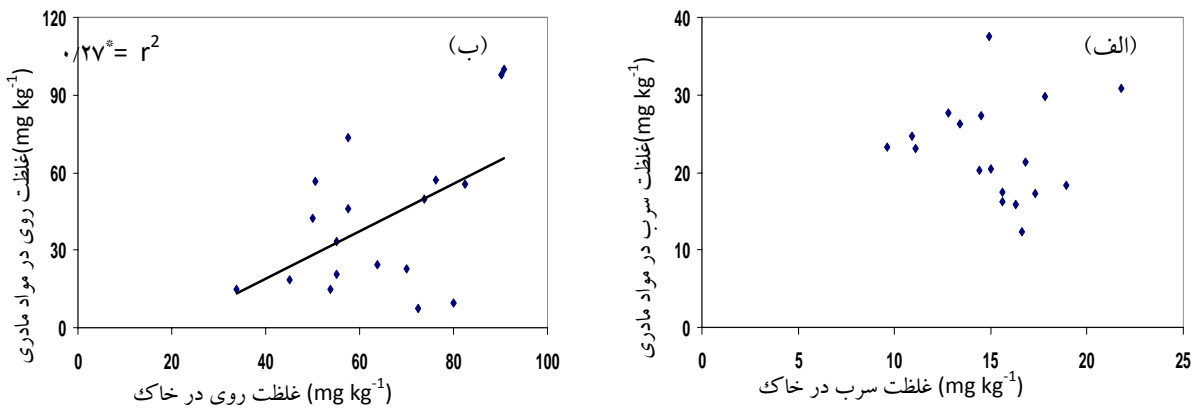
(شکل ۷) - نمودار همبستگی غلظت سرب کل (الف) و روی کل (ب) در خاک و مواد مادری
