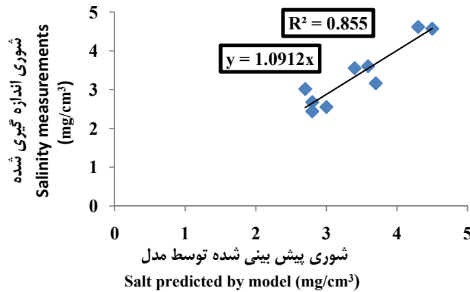
شکل ۳- نتایج صحت سنجی مدل SWAP در توزیع شوری
