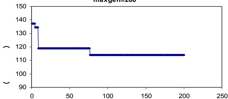
شکل ۲- روند تغییرات تابع هدف در رژیم جریان ثابت در برابر شماره نسل در شرایط بدون گیاه
