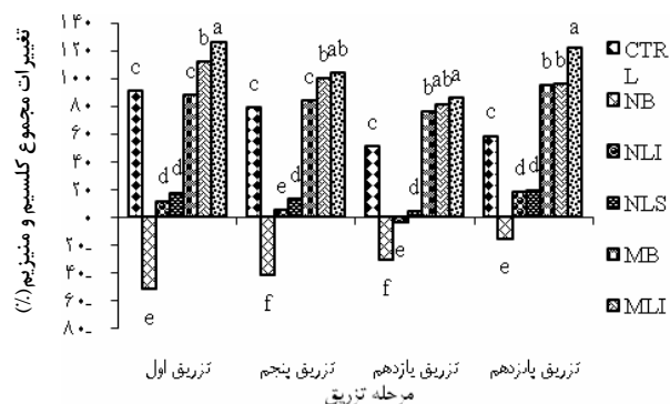
شکل ۹- درصد تغییرات مجموع کلسیم و منیزیم پساب در مراحل مختلف تزریق
