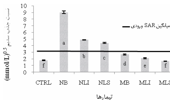
شکل ۱۰- میانگین SAR پساب خروجی در کل دوره
