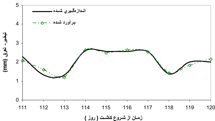
(شکل ۵)- تبخیر- تعرق خیار گلخانه‌ای در مرحله انتهایی رشد (معادله ۱۲)
