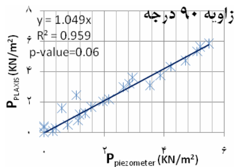
شکل ۸ و ۹- مقایسه داده های فشار پیزومتري و PLAXIS، در زوایای ۶۰ و ۹۰ درجه
