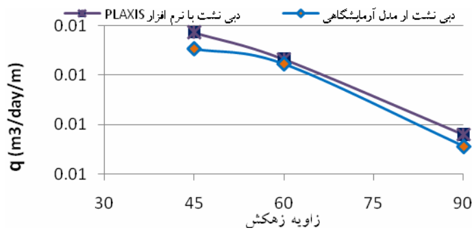
شکل ۱۵- دبی نشت از مدل آزمایشگاهی و PLAXIS در شاخص (p/h)^3
