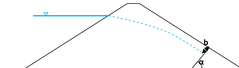
شکل ۱۲- نمای شماتیک از مدل و محل عبور خط فریاتیگ از زهکش پنجه
