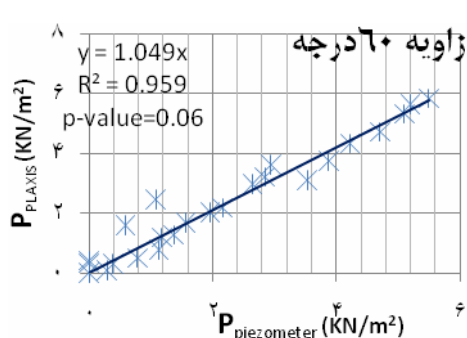
شکل ۸ و ۹- مقایسه داده های فشار پیزومتري و PLAXIS، در زوایای ۶۰ و ۹۰ درجه
