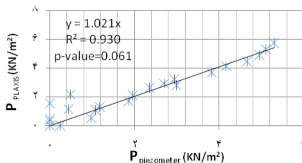
شکل ۱۰- مقایسه داده های فشار پیزومتري و PLAXIS، زاویه زهکش پنجه ۴۵ درجه
