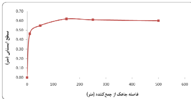
شکل ۸- شعاع تأثیر جمع‌کننده مزرعه مورد مطالعه
