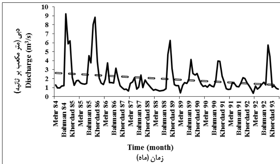
شکل ۶- هیدروگراف رودخانه الشتر در محل ایستگاه کهمان در بالادست
