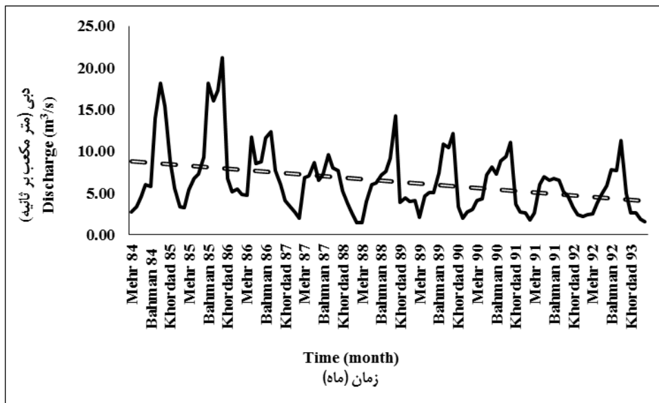
شکل ۷- هیدروگراف رودخانه الشتر در محل ایستگاه هیدرومتری سراب صیدعلی در پایین‌دست
