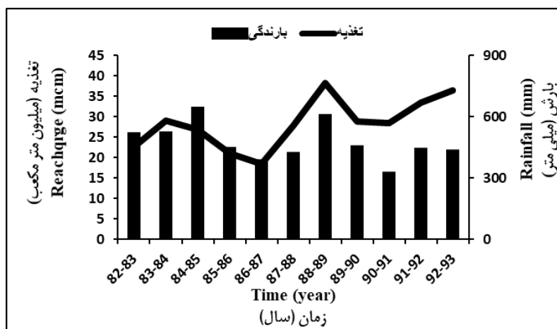
شکل ۵- سری زمانی مقدار بارش و تغذیه به آبخوان الشتر (محاسبه شده به روش نوسان سطح ایستابی)
