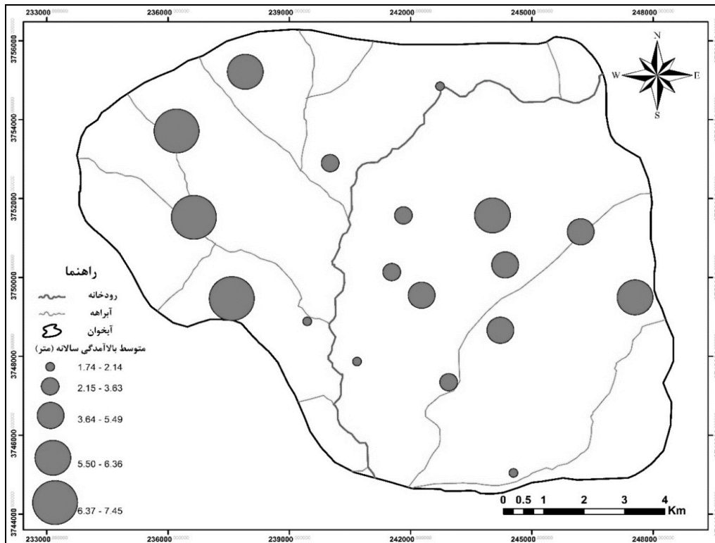
شکل ۴- متوسط بالآمدگی سالانه سطح ایستابی در دوره تغذیه در پیزومترهای آبخوان الشتر Figure 4-The average annual rise of water table in piezometers of the Aleshtar aquifer during the recharge period
