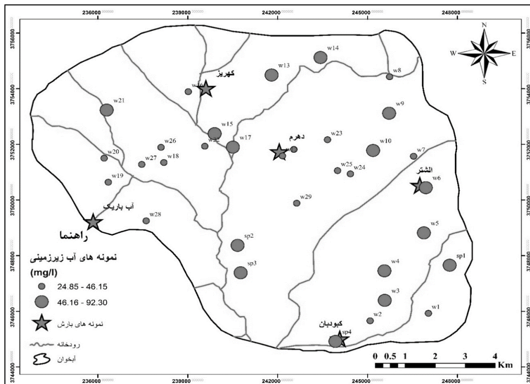
شکل ۹- تغییرات مکانی غلظت کلر آب زیرزمینی در محدوده آبخوان الشتر Figure 9- Spatial variations of groundwater chloride concentration in Aleshtar aquifer
