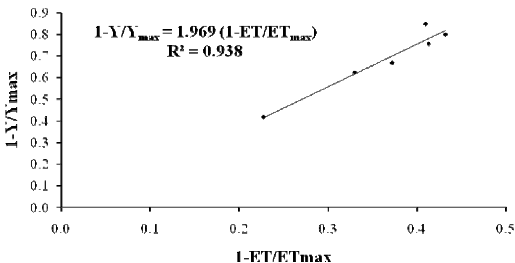
شکل ۴- همبستگی بین افت نسبی عملکرد گوجه‌فرنگی و افت نسبی تبخیر و تعرق
