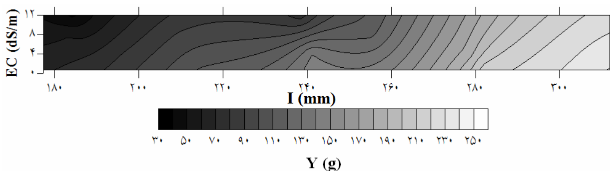
شکل ۳- منحنی‌های هم محصول در شرایط تنش توأمان شوری و خشکی
