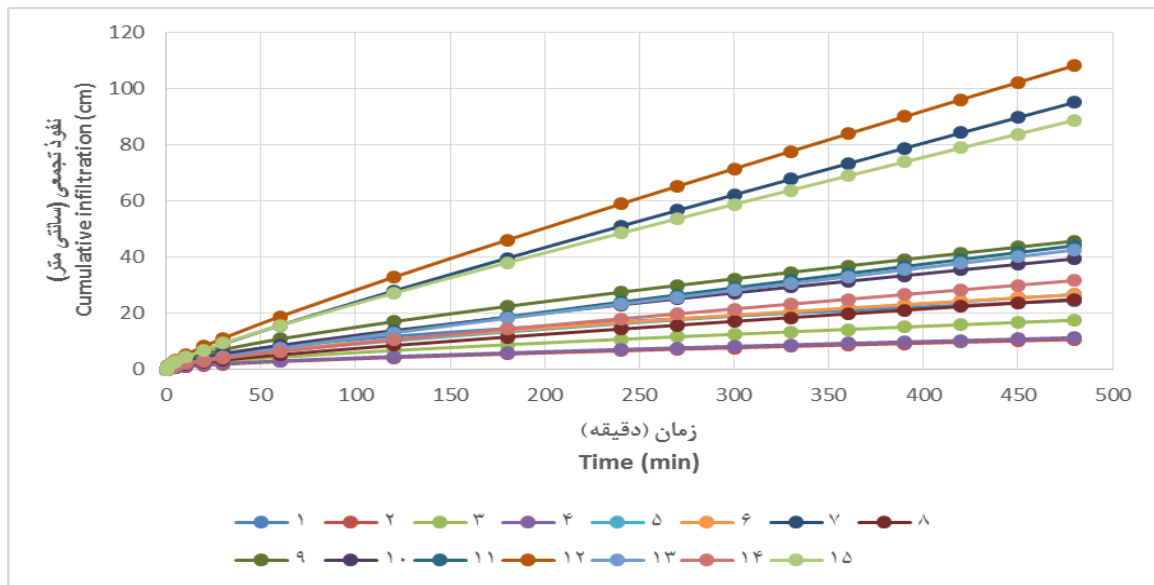
شکل ۷- منحنی نفوذ تجمعی برای ۱۵ نمونه از داده‌های مهرابی و سپاسخواه Figure 7- Cumulative infiltration curves of 15 sites over Mehrahi and Sepaskhah data
