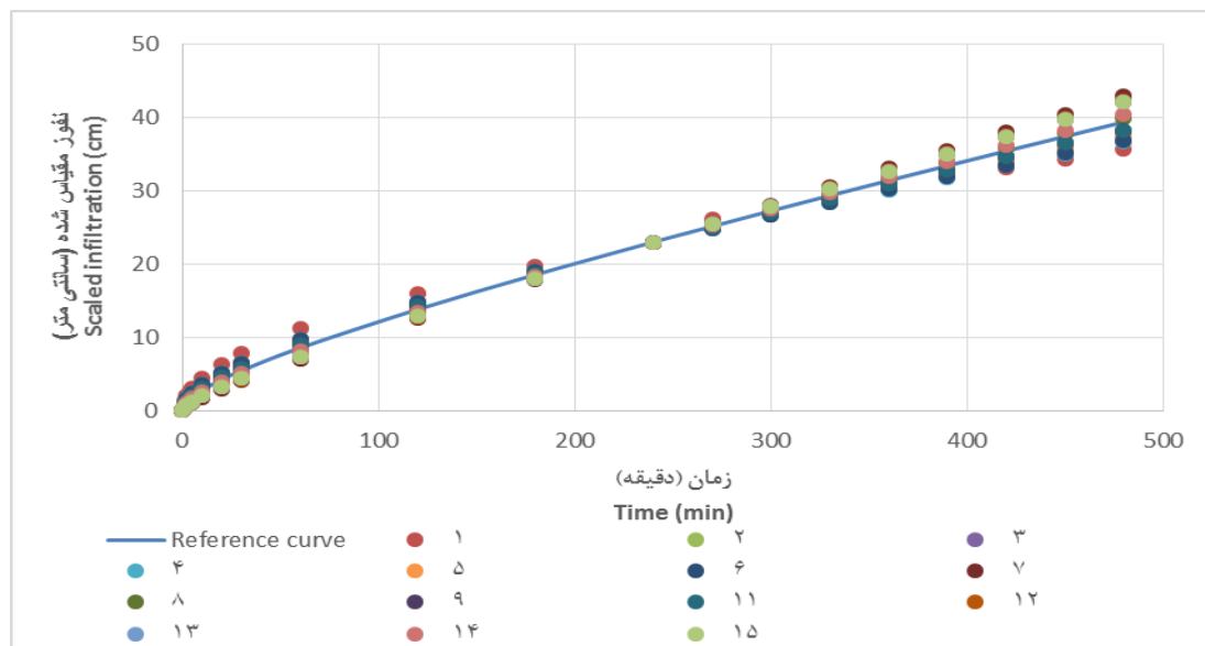
شکل ۸- منحنی نفوذ مقیاس شده تجمعی برای ۱۵ نمونه از داده‌های تحقیق مهرابی و سپاسخواه Figure 8- Scaled cumulative infiltration curves of 15 sites over Mehrahi and Sepaskhah data
