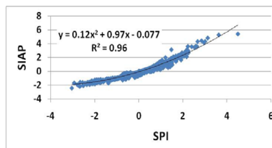
شکل ۴- همبستگی بین دو نمایه SPI و SIAP در مقیاس زمانی فصلی
