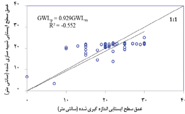
شکل ۵- مقایسه سطح ایستابی اندازه‌گیری و برآورد شده توسط مدل
