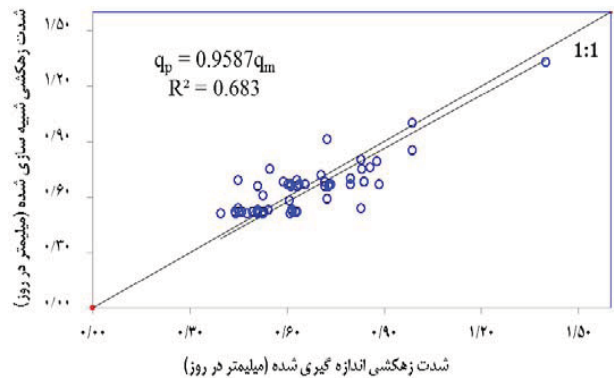
شکل ۶- مقایسه شدت زهکشی اندازه‌گیری و برآورد شده توسط مدل
