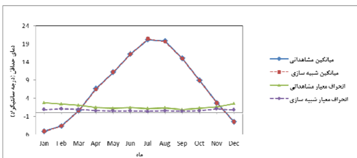
شکل ۳- میانگین و انحراف معیار مقادیر مشاهداتی و شبیه‌سازی شده دمای حداقل ماهانه
