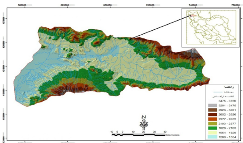
شکل ۱- نقشه DEM حوضه آبریز آبی‌چای
