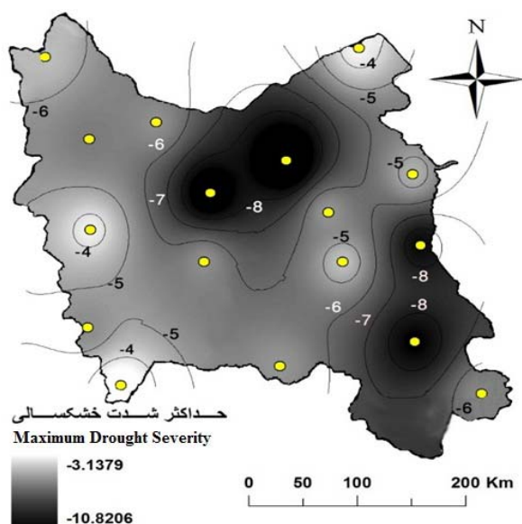
شکل ۱۱- منحنی‌های هم رقوم max severity منطقه با دوره بازگشت ۱۰ سال Figure 11- Equivalent Curve of Max Drought Severity of Study Area with 10 Years of Return Peiod
