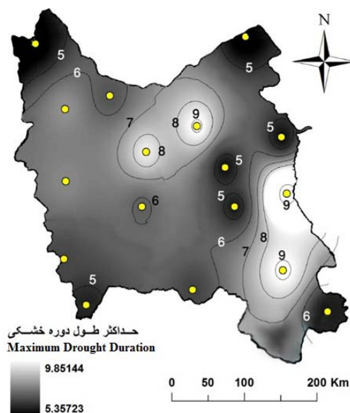
شکل ۱۲- منحنی‌های هم رقوم max duration با دوره بازگشت ۱۰ سال Figure 12- Equivalent Curve of Max Drought Duration of Study Area with 10 Years of Return Peiod
