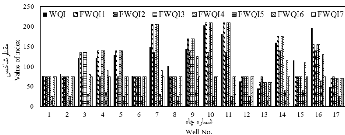
شکل ۳- مقادیر WQI و FWQI برای شهریور ماه سال ۱۳۸۴ Figure 3- WQI and FWQI (September 2005)
