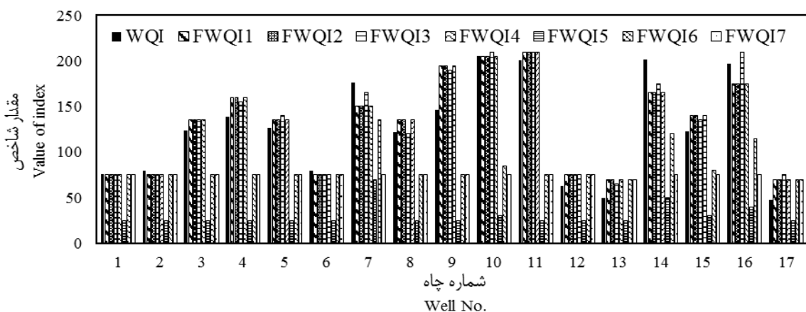
شکل ۵- مقادیر WQI و FWQI برای شهریور ماه سال ۱۳۸۵ Figure 5- WQI and FWQI (September 2006)
