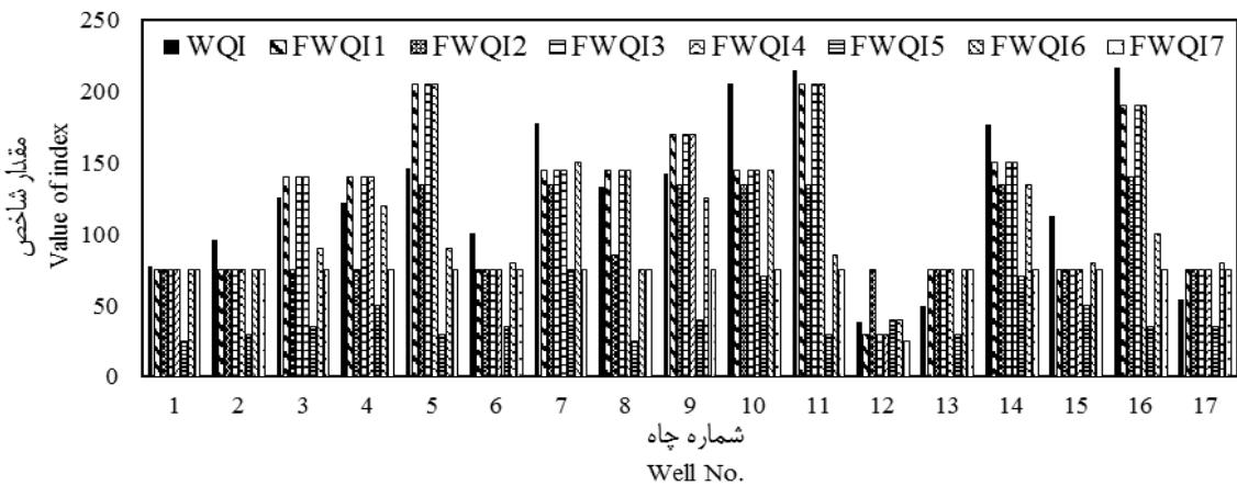
شکل ۲- مقادیر WQI و FWQI برای اردیبهشت ماه سال ۱۳۸۴ Figure 2- WQI and FWQI (May 2005)
