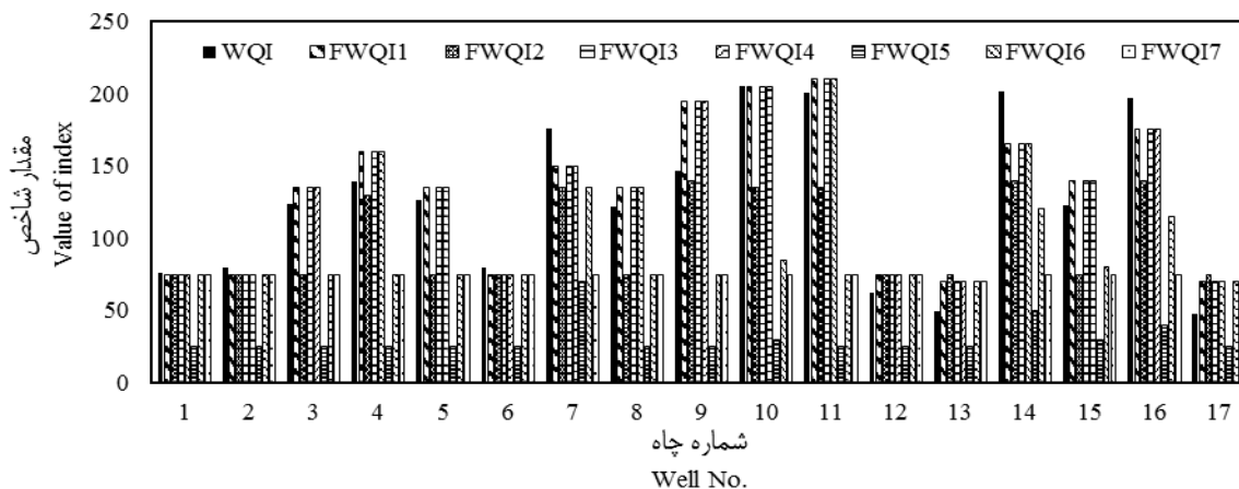
شکل ۴- مقادیر WQI و FWQI برای اردیبهشت ماه سال ۱۳۸۵ Figure 4- WQI and FWQI (May 2006)
