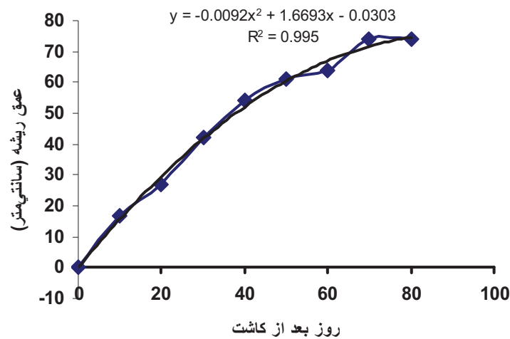
شکل ۱- توسعه عمق ریشه در روزهای بعد از کشت
