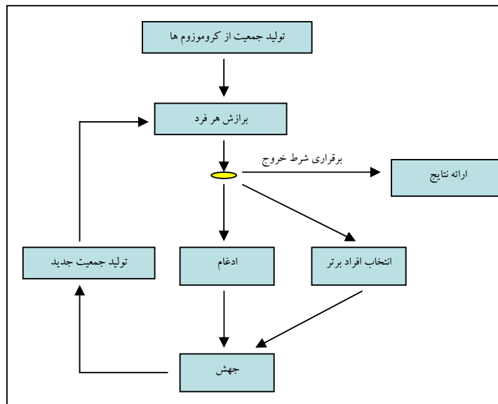
شکل ۲- فلوجارت الگوریتم ژنتیک
