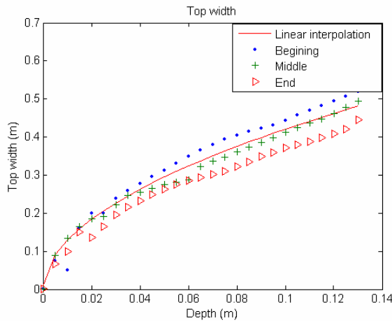
(شکل ۶) - عرض بالایی جویچه نسبت به عمق برای مزرعه رودشت، خط ممند بیانگر متوسط برای سه مقطع، ابتدا، وسط و انتهای جویچه است
