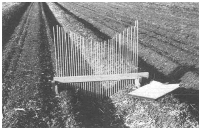
(شکل ۱) - دستگاه مقطع سنج جویچه (۱)
