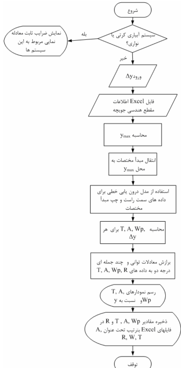
(شکل ۵) - نمودار گردش کار برنامه رایانه‌ای
