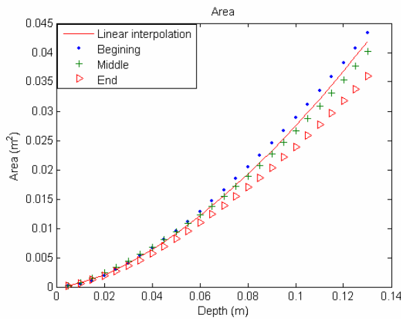
(شکل ۷) - سطح مقطع جویچه نسبت به عمق برای مزرعه رودشت، خط ممند بیانگر متوسط برای سه مقطع، ابتدا، وسط و انتهای جویچه است
