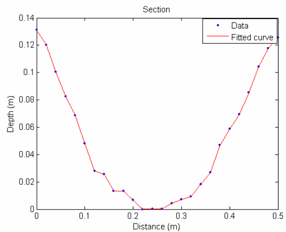
(شکل ۹) - سطح مقطع متوسط جویچه برای مزرعه رودشت، نقاط مربوط به اعداد خوانده شده از دستگاه مقطع سنج جویچه و خط ممند درونیایی خطی برنامه می باشد
