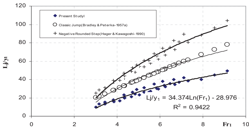
شکل ۸- تغییرات طول بی‌بعد پرش هیدرولیکی در برابر عدد فرود اولیه
