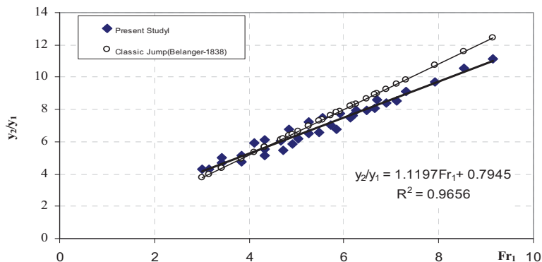
شکل ۵- تغییرات عمق نسبی پرش هیدرولیکی در بستر زبر و صاف به ازای عدد فرود اولیه
