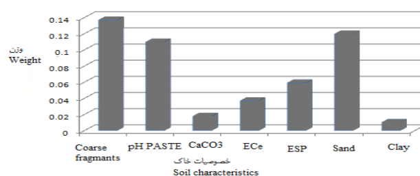
شکل ۲- وزن‌های محاسبه‌شده ویژگی‌های خاک به روش شبکه عصبی با یک نرون
