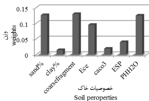
شکل ۳- وزن‌های محاسبه‌شده ویژگی‌های خاک به روش شبکه عصبی با چهار نرون
