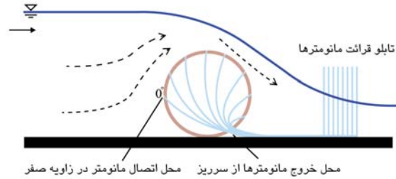
(شکل ۱) - استقرار مانومترها بر روی سرریز در زوایای ۰ تا ۲۱۰ درجه
