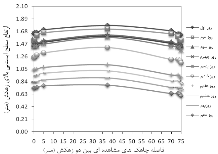
شکل ۴- منحنی سطح ایستابی بین دو زهکش به دنبال کاربرد دومین آبیاری به ترتیب از بالا به پایین در تیمارهای FD، CD 90 و CD 70
