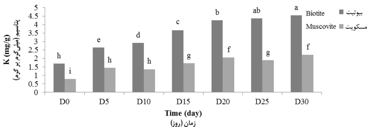
شکل ۳- اثر متقابل زمان و کانی بیوتیت و موسکویت در آزاد سازی پتاسیم
