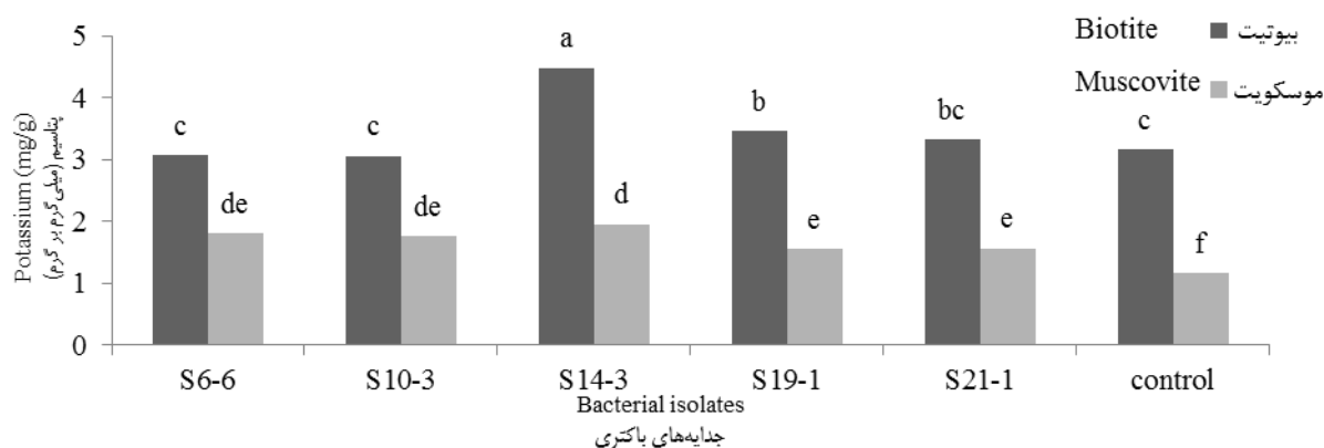
شکل ۲- اثر متقابل ۵ جدایه کارآمد با کانی بیوتیت و موسکویت در آزاد سازی پتاسیم
