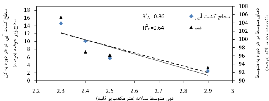
شکل ۱۲- همبستگی بین تغییرات سطح کشت آبی و دما متوسط سالانه با دبی متوسط سالانه قشلاق امیر
